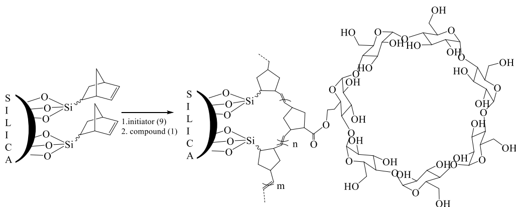
Рисунок 50 – Схема закрепления CD-нов на поверхности кремнезёма [15]
