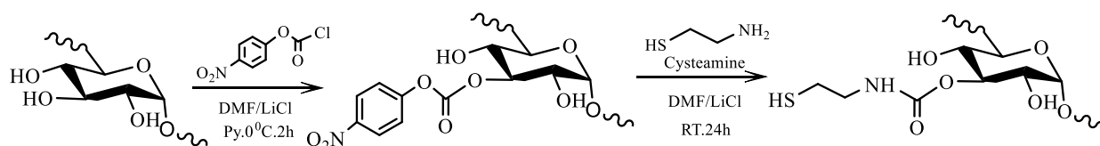
Рисунок 16 – Двухстадийный синтез тиолированного декстрана [18]
