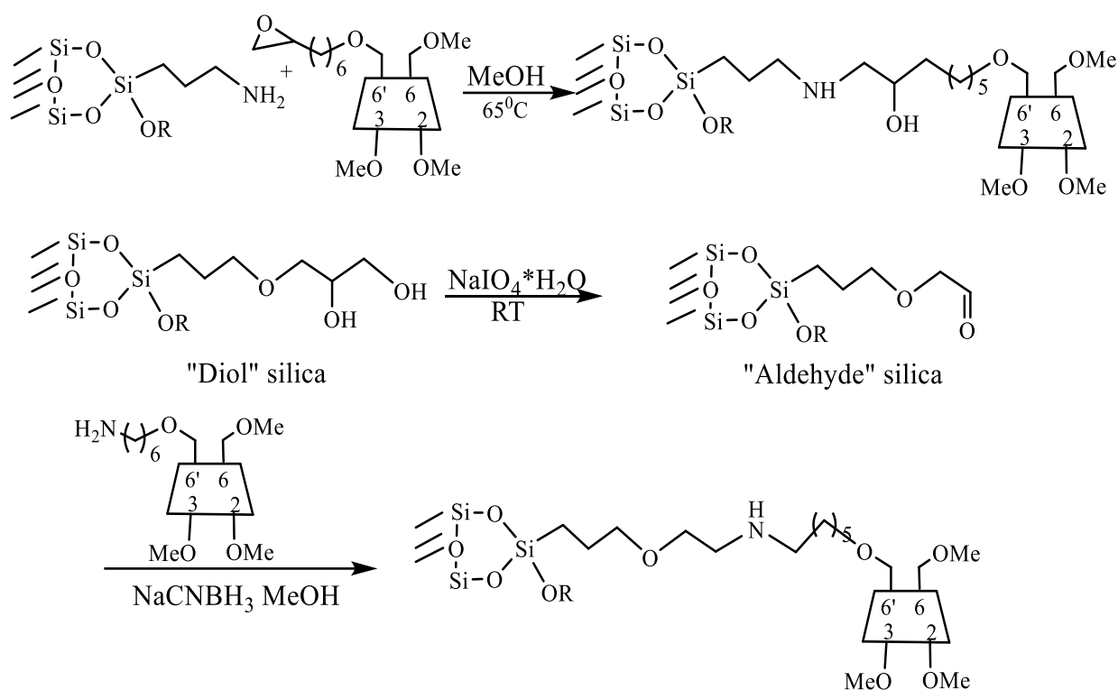
Рисунок 6 – Модификация поверхности кремнезёмов производными CD-нов [14]
