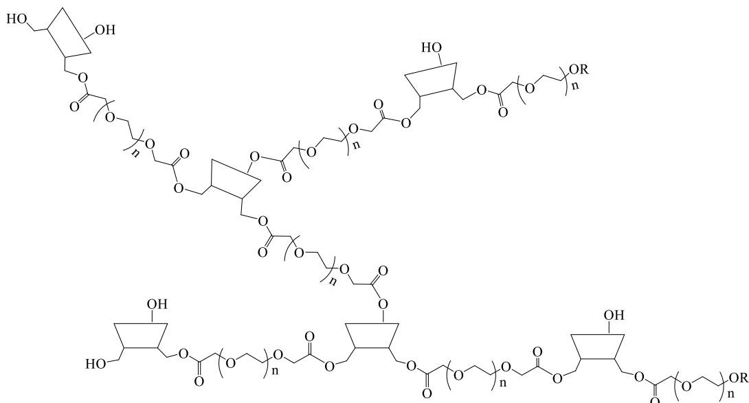
Рисунок 12 – Строение CD-содержащих полимеров на основе ПЭГ [16]
