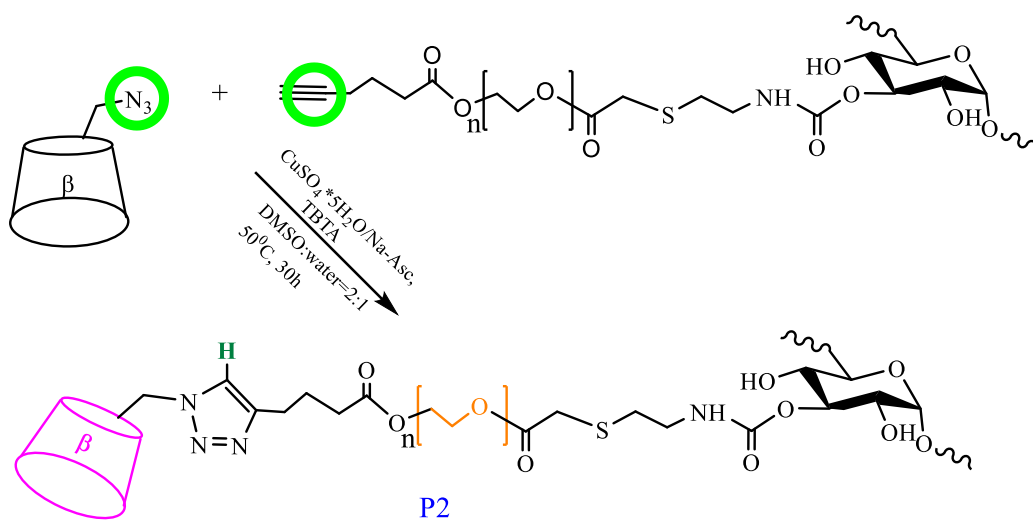
Рисунок 19 – Реакционный маршрут для азид-замещенных \beta -CD-нов [18]
