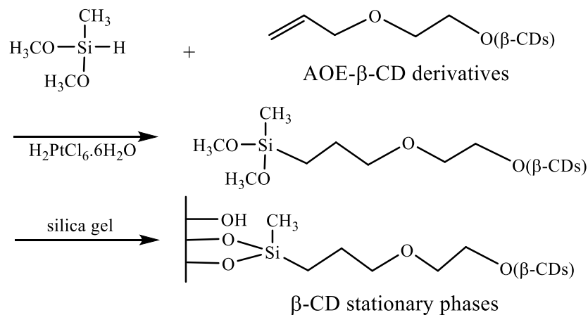
Рисунок 5 – Модификация кремнезема \beta -CD-ом и его производными [13]
